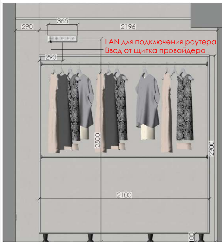
Развёртка стены мастер гардероба №12
