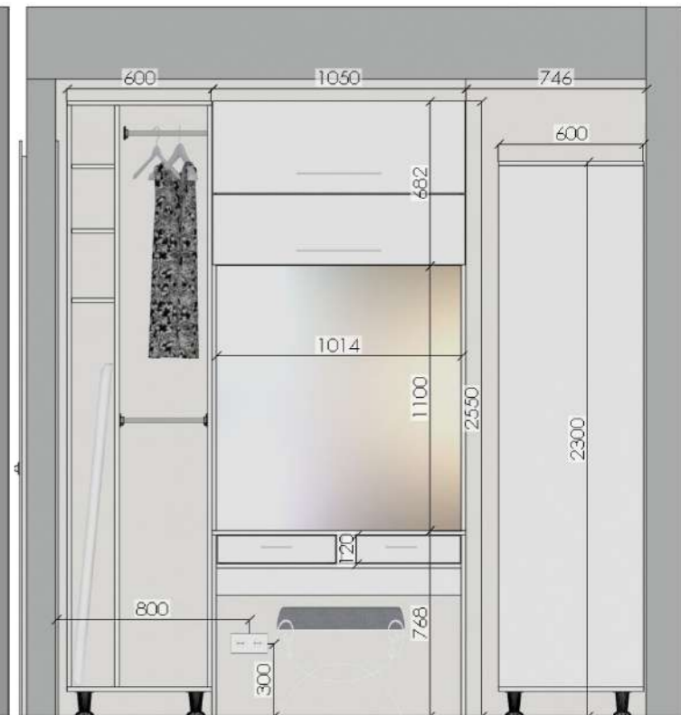
Развёртка стены мастер санузла №15
