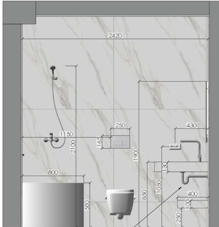
Развёртка стены мастер санузла №8
