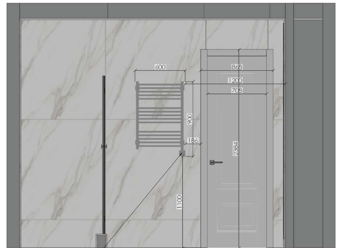
Развёртка стены гостевого санузла №17
