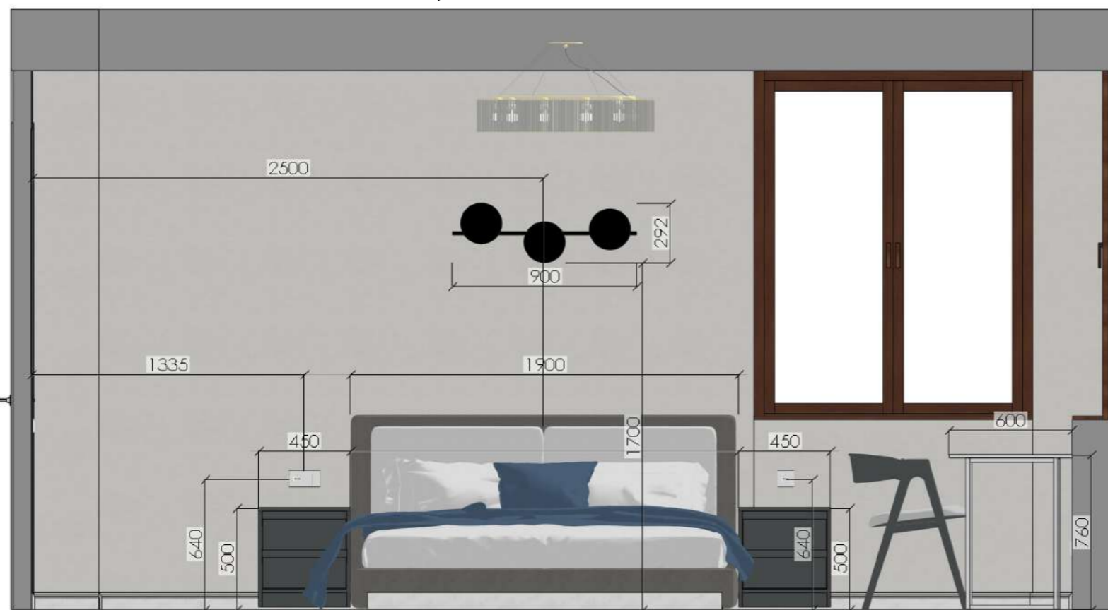
Развёртка стены спальни №4
