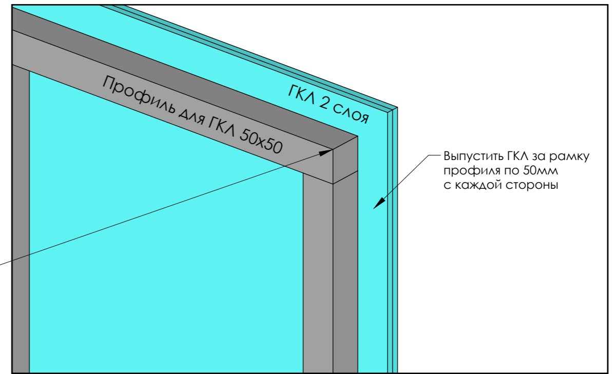
Вид конструкции с задней стороны
