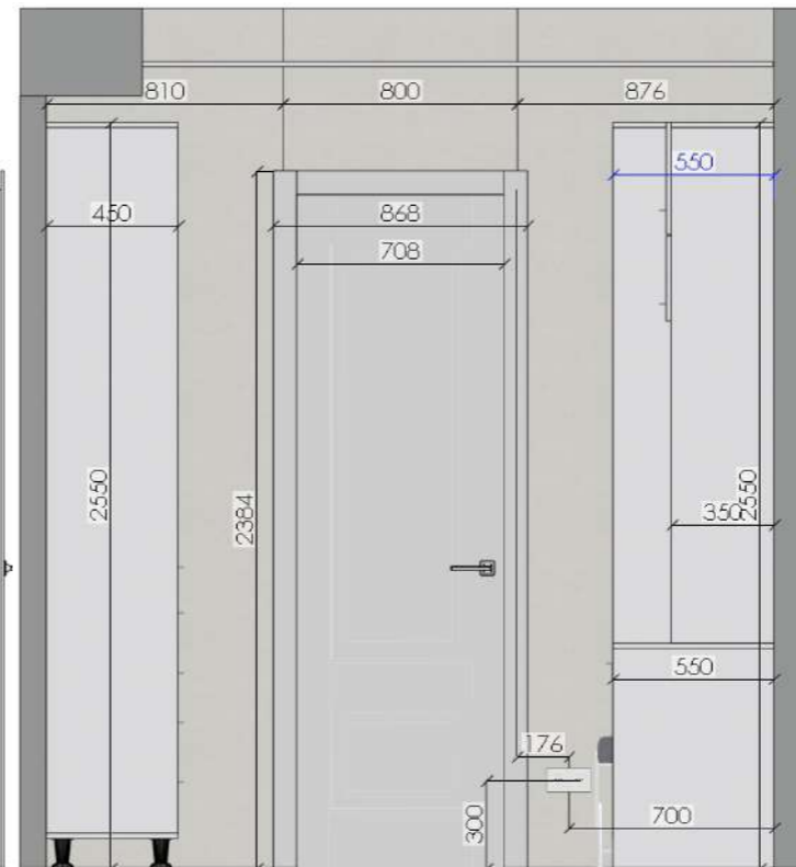
Развёртка стены мастер санузла №14
