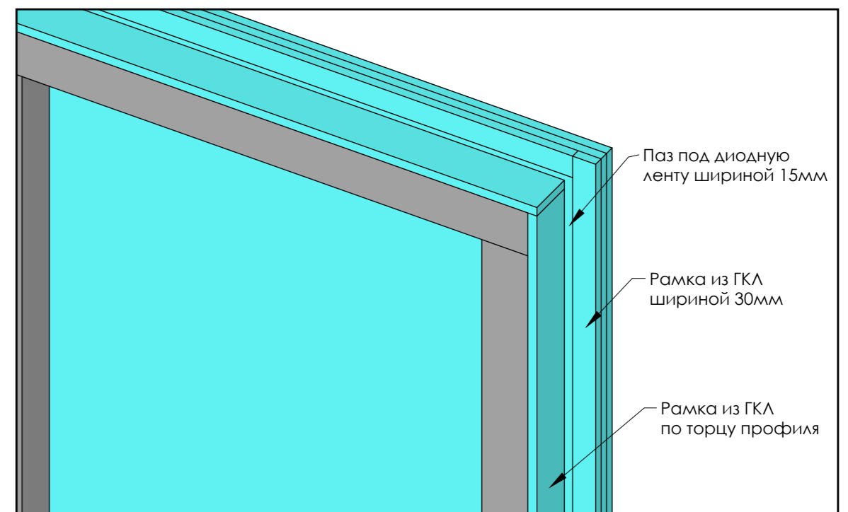
Финишный вид конструкции с задней стороны
