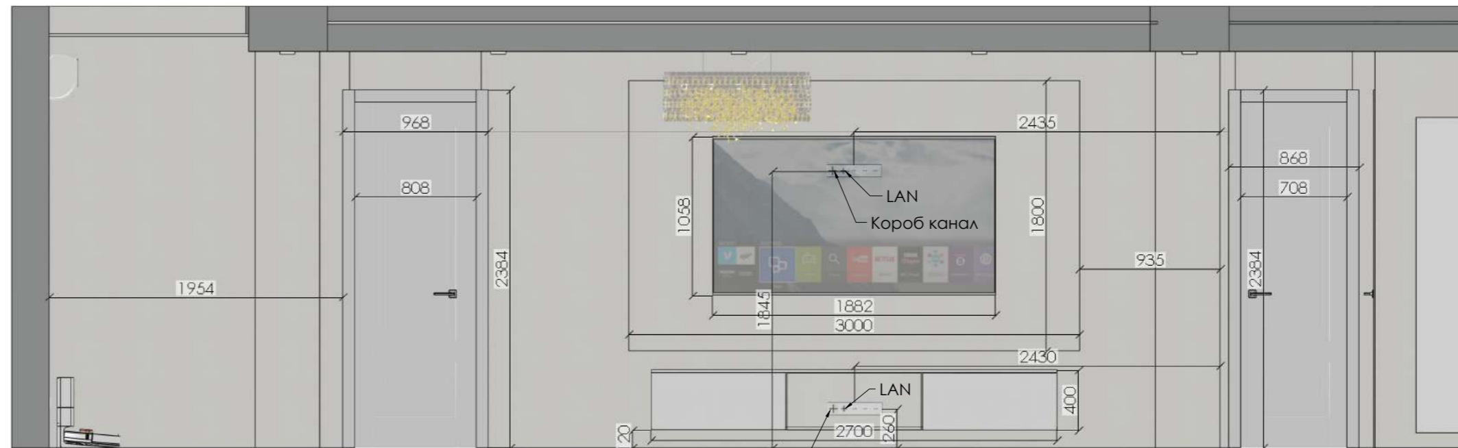
Развёртка стены кухни - столовой №28
