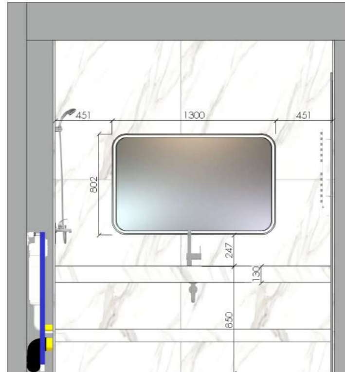
Развёртка стены мастер санузла №9
