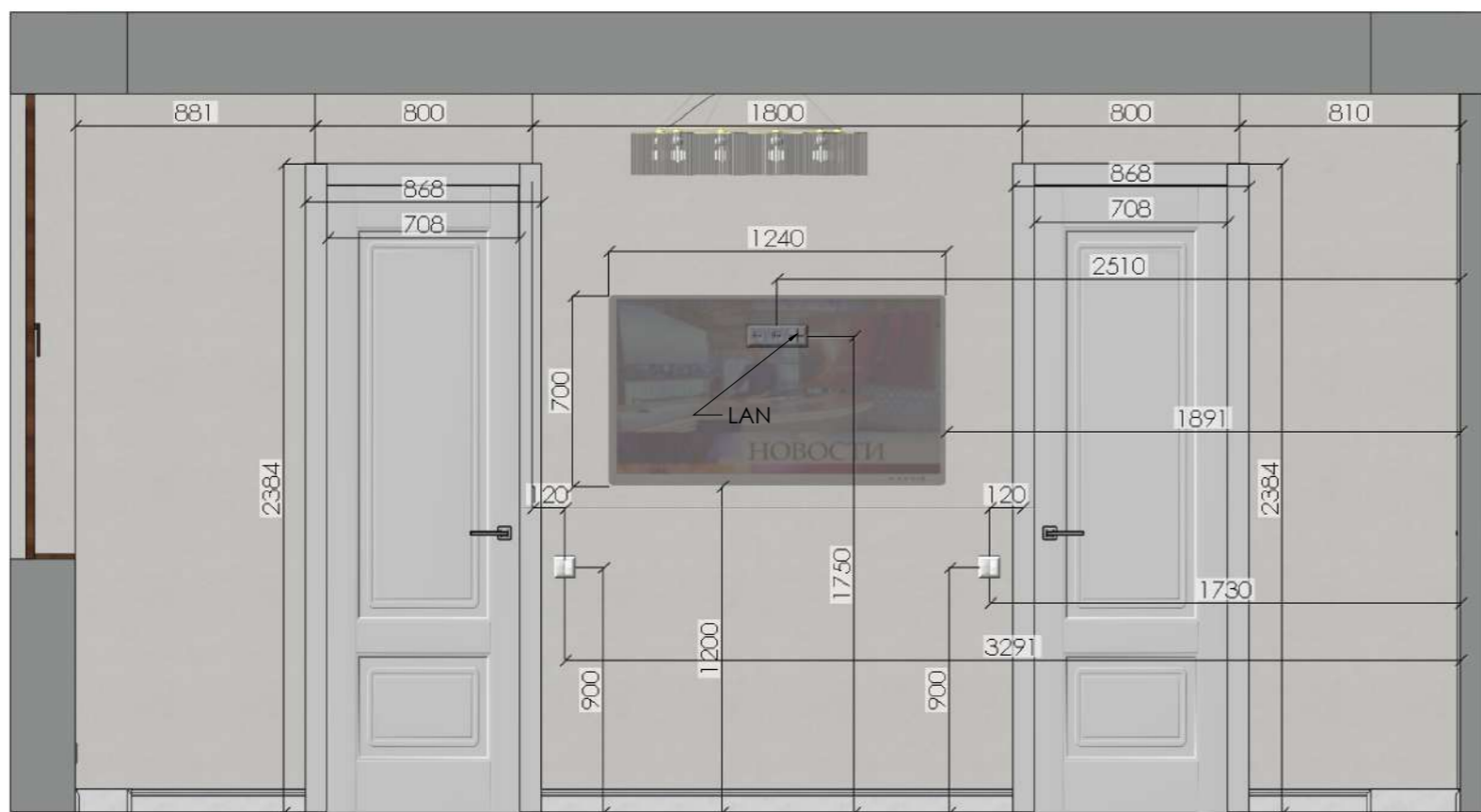
Развёртка стены спальни №6
