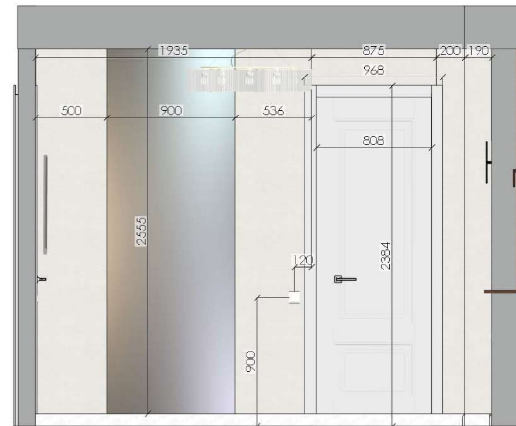
Развёртка стены спальни №7
