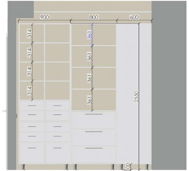
Развёртка стены гардероба в детской №26
