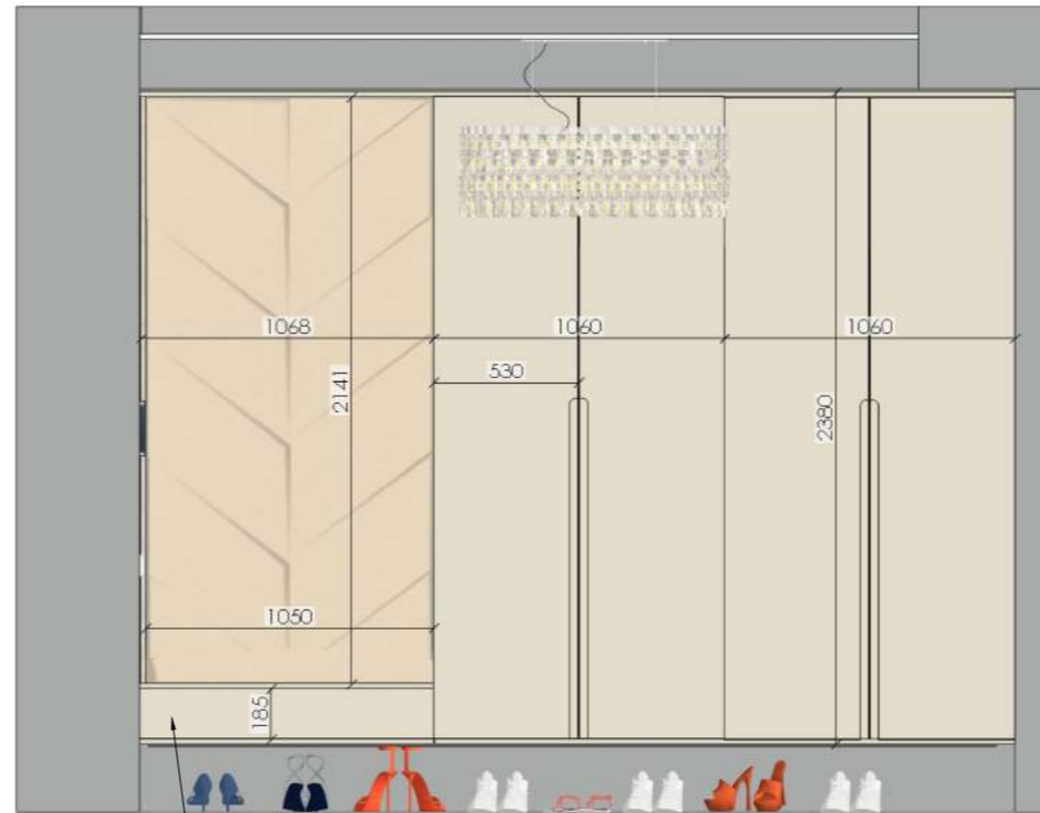
Развёртка стены коридора №19
