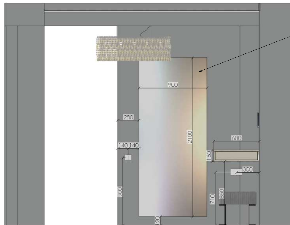
Развёртка стены коридора №21
