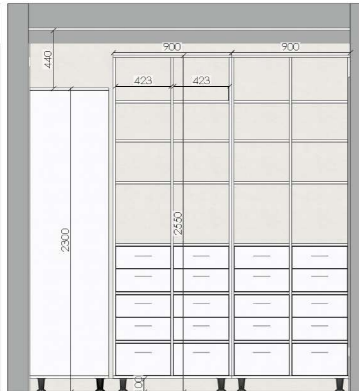
Развёртка стены мастер санузла №13
