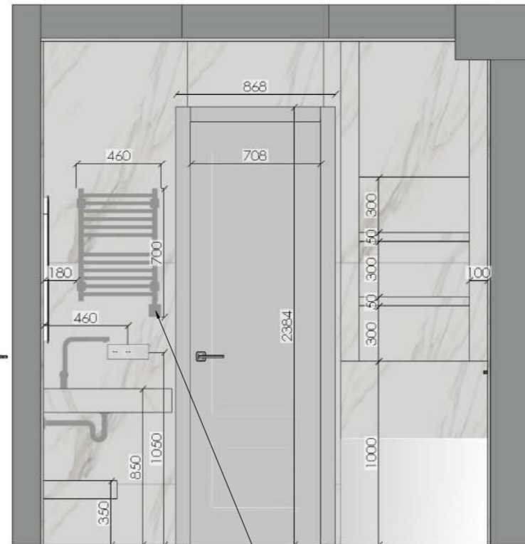
Развёртка стены мастер санузла №10
