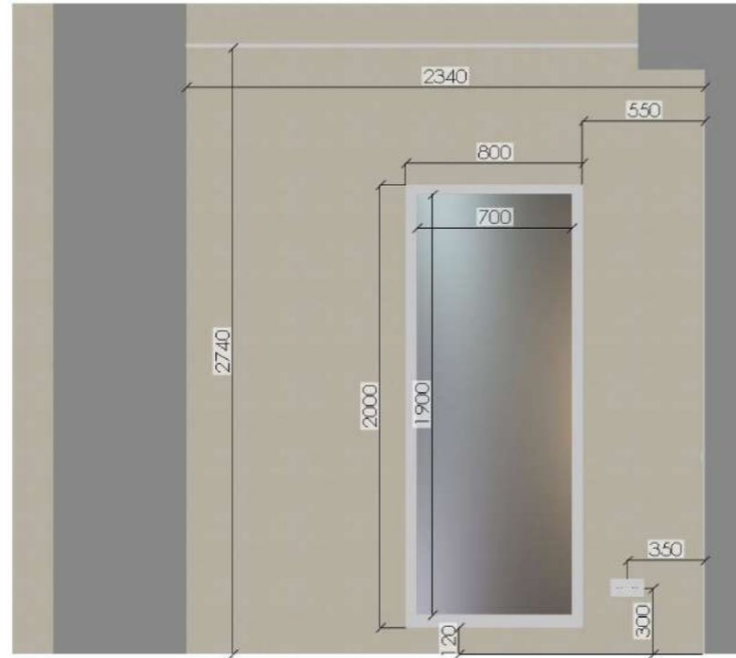
Развёртка стены гардероба в детской №24
