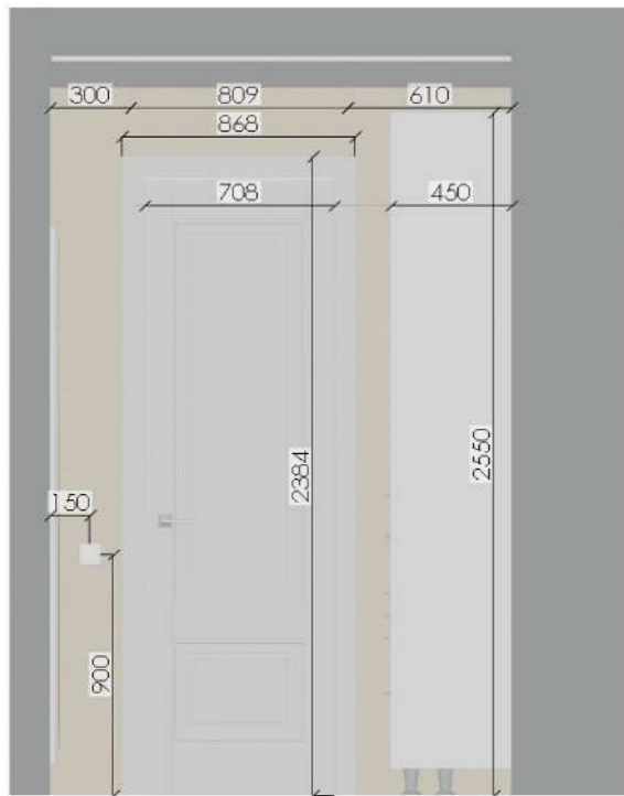
Развёртка стены гардероба в детской №23
